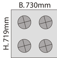
Mod. 2: Kondensator 4 Lüfter
