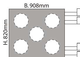
Mod. 2: Kondensator 5 Lüfter
