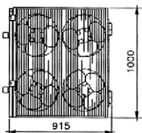
Mod. 5: Kondensator 4 Lüfter
