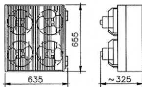
Mod. 6: Kondensator 4 Lüfter
