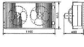
Mod. 2: Kondensator 2 Lüfter
