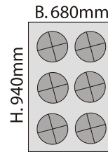
Mod. 4: Kondensator 6 Lüfter
