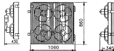
Mod. 4: Kondensator 4 Lüfter
